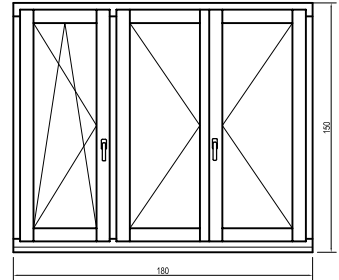
Háromszárnyas: bukó-nyíló + középen felnyíló (tokosztós)
