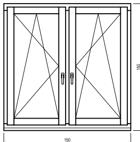
Bukó-nyíló + bukó-nyíló (tokosztós)
