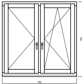
Oldalt nyíló + bukó-nyíló (tokosztós)
