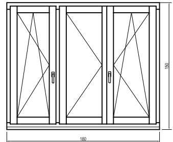
Háromszárnyas: bukó-nyíló + középen felnyíló bukó-nyíló (tokosztós)
