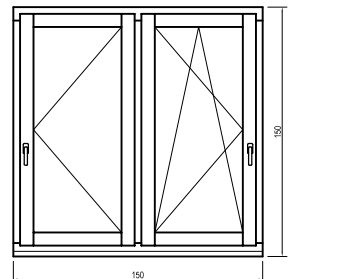
Középre nyíló: oldalt nyíló + bukó-nyíló (tokosztós)
