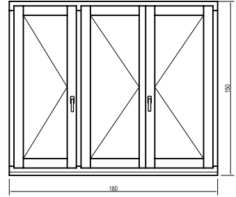
Háromszárnyas: oldalt nyíló + középen felnyíló (tokosztós)
