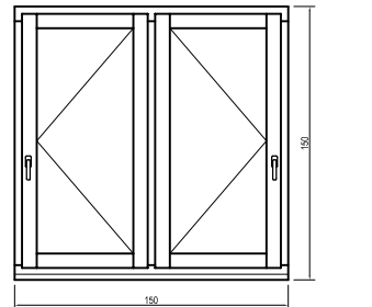
Középre nyíló: oldalt nyíló + oldalt nyíló (tokosztós)
