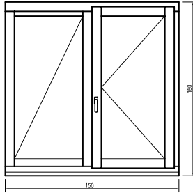
Fix + oldalt nyíló (tokosztós)
