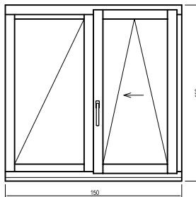
Fix + bukó-toló (tokosztós)
