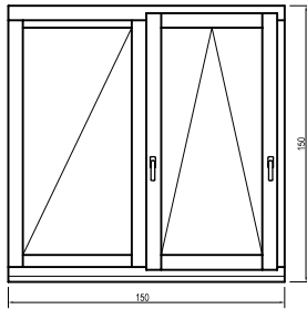
Fix + bukó (kétkilincses, tokosztós)
