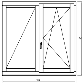
Fix + bukó-nyíló (tokosztós)
